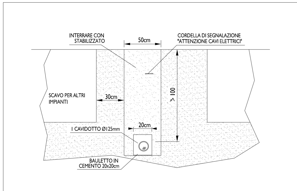
PARTICOLARE SCAVO SOTTO LA STRADA - SCALA 1:20
