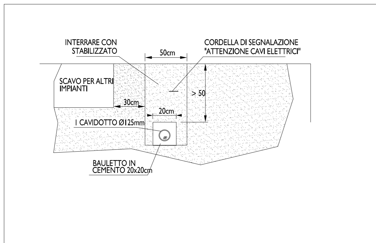
PARTICOLARE SCAVO SOTTO LA PISTA CICLABILE SCALA 1:20
